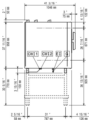
Zij aanzicht
